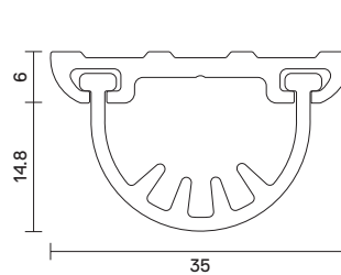
AAS3503 (BLADES IN) ↑
