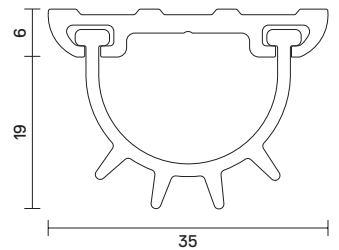
AAS3503 (BLADES OUT) ↑
